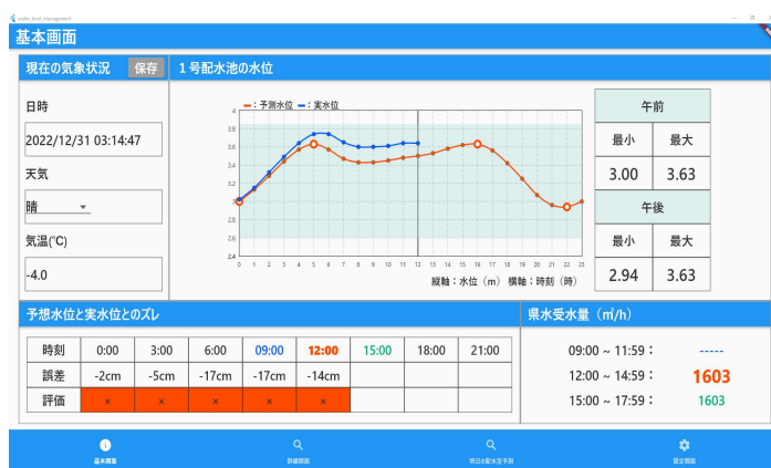
図2. 水位調整アプリ画面
